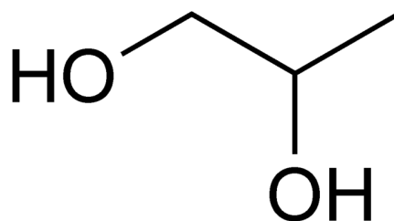
FIGURE 9 : FORMULE CHIMIQUE DU PROPYLENE GLYCOL
