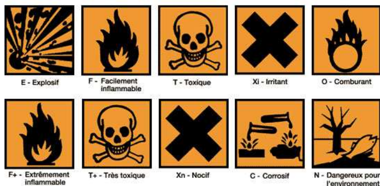
FIGURE 65 : PICTOGRAMMES DE DANGER, LISTES DES MENTIONS DE DANGER ET CONSEILS DE PRUDENCE SUR LE RISQUE CHIMIQUE UTILISÉS ACTUELLEMENT(SOURCE : INRS)
